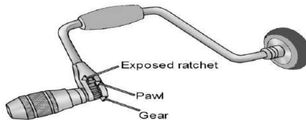
Fig. 4.19: Ratchet Brace
